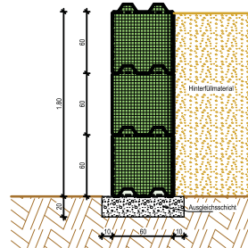
Pos. 1.4.3 - Betonstein 80
