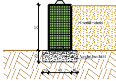
Pos. 1.3.1 - Betonstein 60
