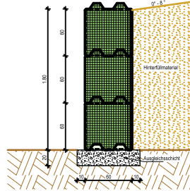
Pos. 2.4.3 - Betonstein 80
