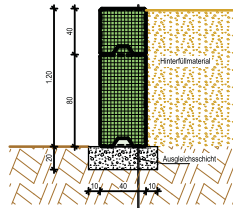
Pos. 1.3.2 - Betonstein 60
