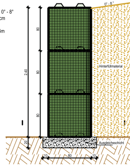
Pos. 2.4.3 - Betonstein 80
