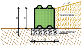
Pos. 2.4.1 - Betonstein 80
