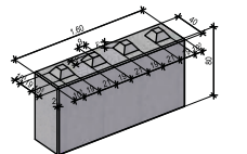
Betonbaustein 160/80/40 cm ca. 1.200 kg
