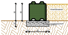
Pos. 1.4.1 - Betonstein 80
