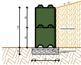
Pos. 2.4.2 - Betonstein 80
