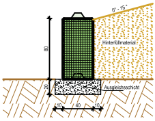
Pos. 2.3.1 - Betonstein 60
