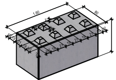
Betonbaustein 160/80/40 cm ca. 1.200 kg
